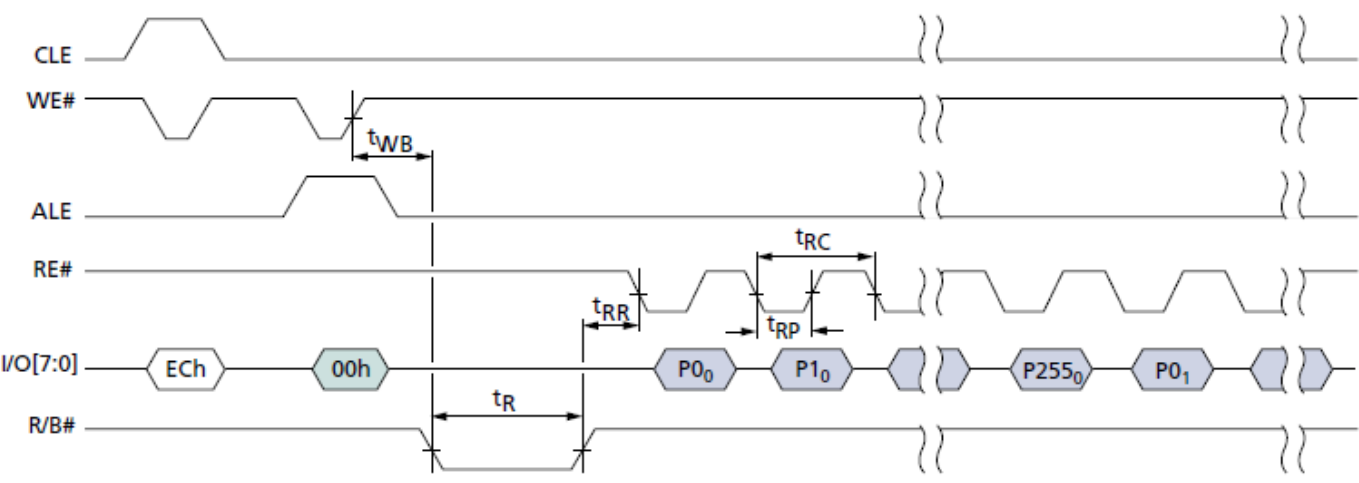
READ PARAMETER PAGE
